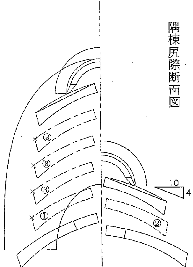
二の鬼際断面図
