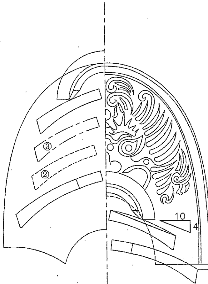
稚児棟尻際断面図
