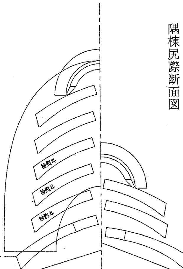
二の鬼際断面図
